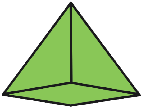
Pyramid
