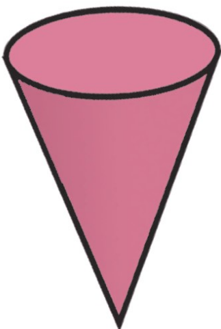
Cone
